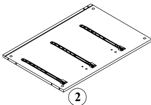
2 # RJ038-010-023-RSP # RJ038-010-024-RSP x1 Right Side Panel x1 Panneau Côté Droite x1 Panel Derecho
