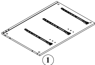
1 # RJ038-010-023-LSP # RJ038-010-024-LSP x1 Left Side Panel x1 Panneau Latéral Gauche x1 Panel Lateral Izquierdo
